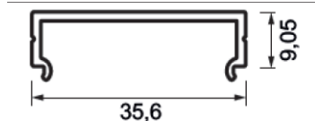
501-563-5#000 Diffuseur PMMA, opale
