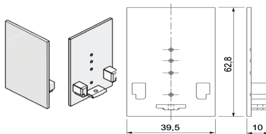
550-573-xx Embout de finition Epic VIII
