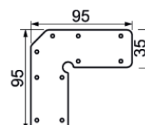
550-564-92 Raccordement d'angle
