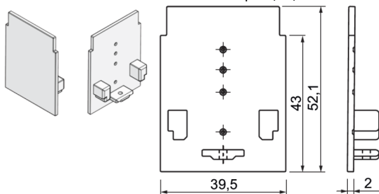
550-567-xx Embout de finition Epic III
