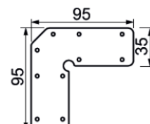
550-564-92 Raccordement d'angle
