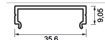
501-563-8#000 Diffuseur PMMA, opale Noir
