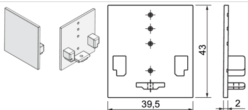
550-566-xx Embout de finition Epic II, IV, V et VI
