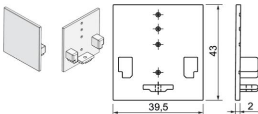
550-566-zz Embout de finition Epic II
