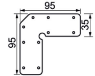
550-564-92 Raccordement d'angle
